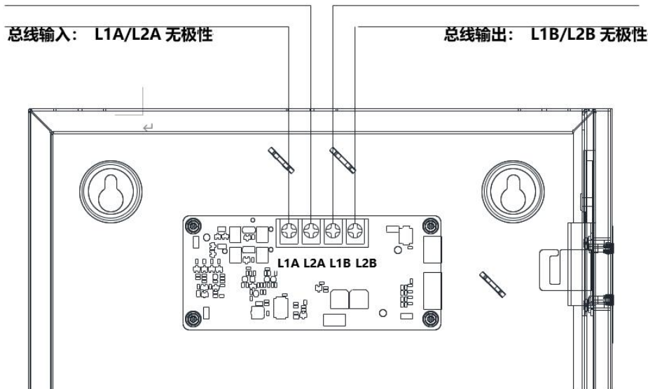
图 2 接线示意图
