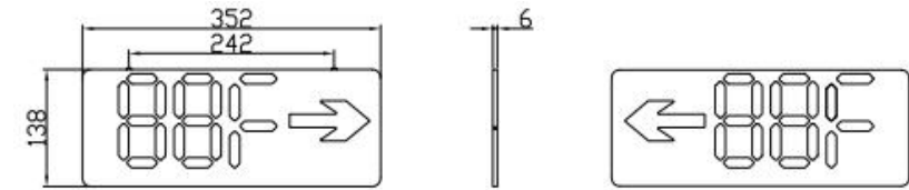
双面外形尺寸示例
