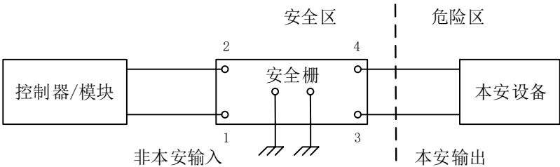
图 3 接线示意图
