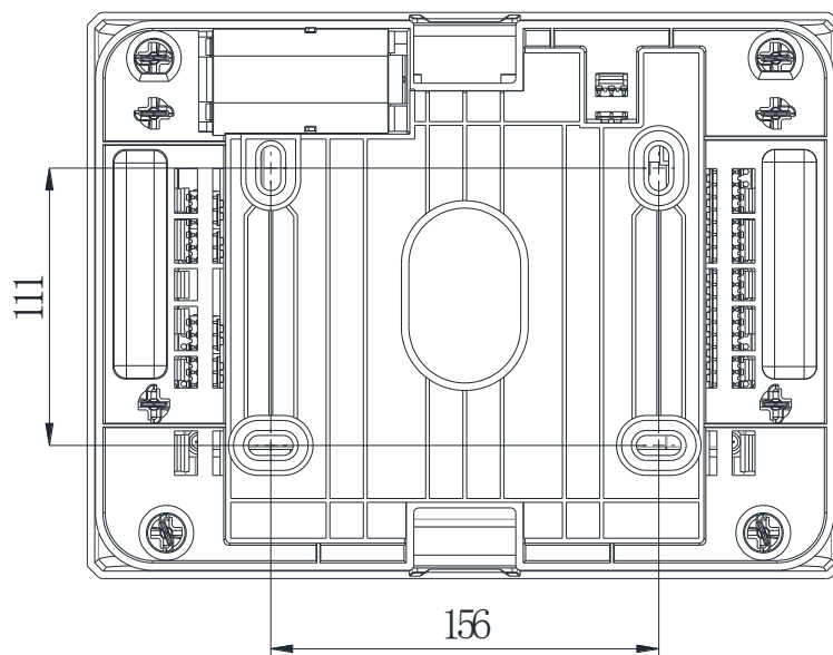
图 2 安装尺寸图
