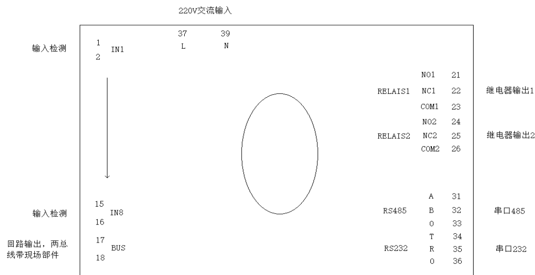
图 3 端子接线图
